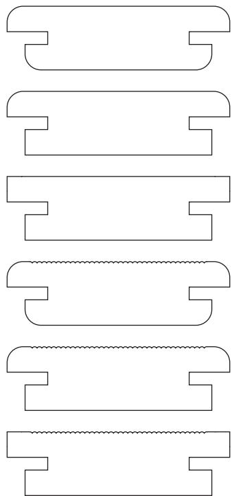
Perfis de usinagem do Deck:
